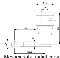
Messeinsatz, radial versetzt mit HM-Kugel \varnothing 5 mm Nr. 5061009
